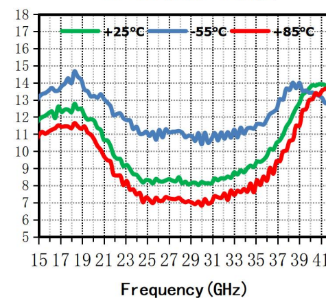
OP-1dB (dBm) vs. 温度
