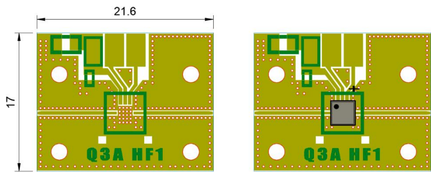
XT4014QP3 评估板
