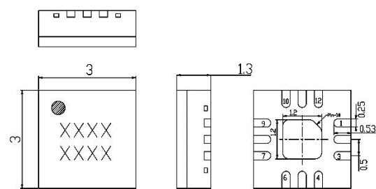
封装外形尺寸( mm)
