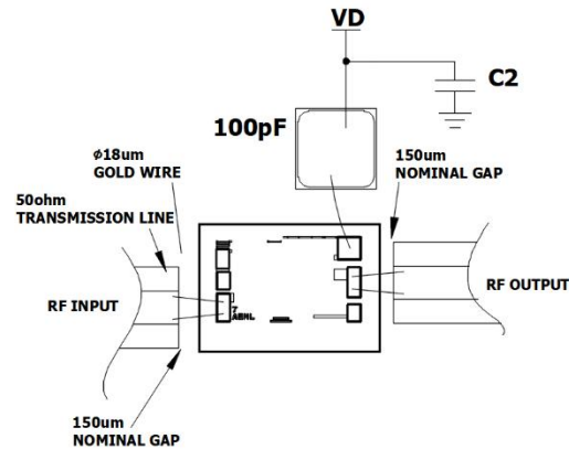
裸芯片推荐装配图
