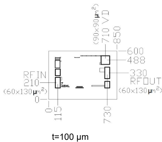
裸芯片外形尺寸( μm)
