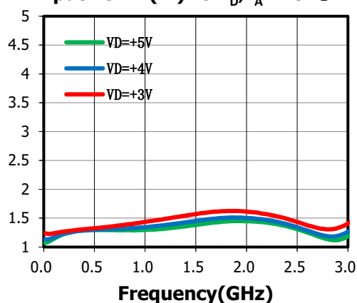
Input VSWR(:1) vs. V_D, T_A=+25^\circ C
