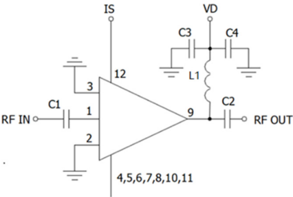
应用电路图
