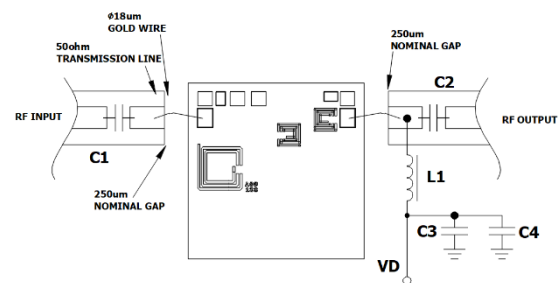
裸芯片推荐装配图
