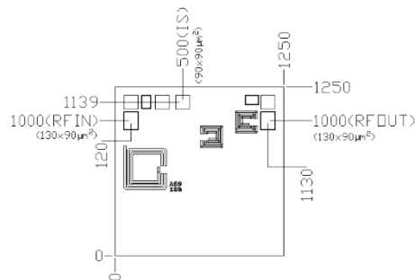
裸芯片外形尺寸( μm)
