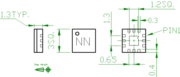
封装外形尺寸( mm)
