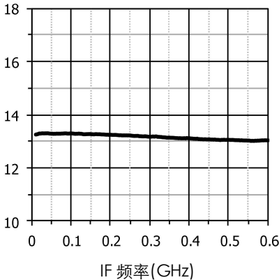
下变频增益(dB)
