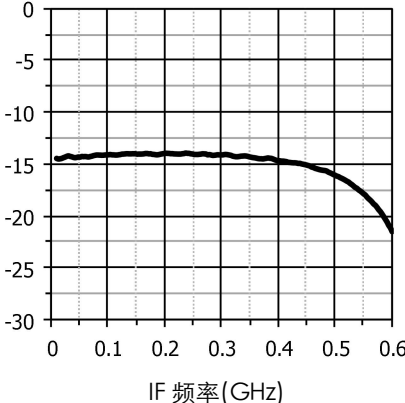
中频端回波损耗(dB)
