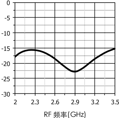
射频端回波损耗(dB)
