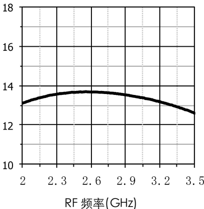
下变频增益(dB)
