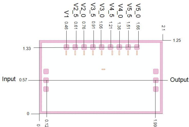
外形和端口尺寸 (mm)
