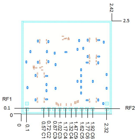
外形和端口尺寸 (mm)
