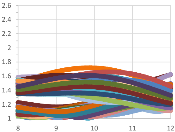
输入驻波比 ( : 1 )
