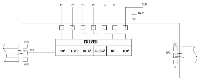
推荐装配图
