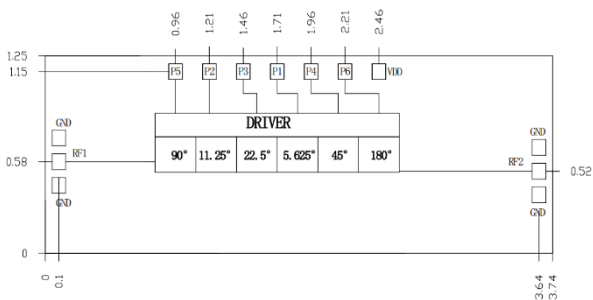
外形和端口尺寸 (mm)
