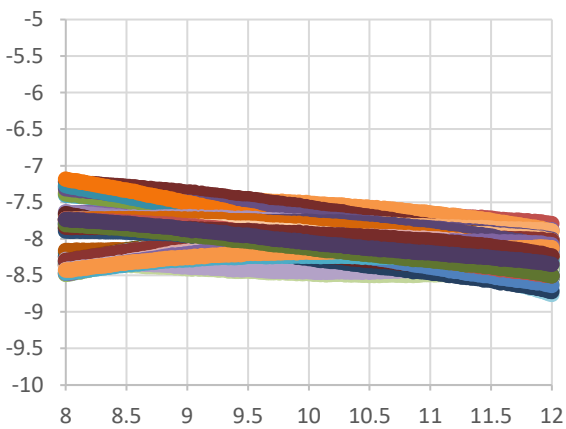
插入损耗 (dB)
