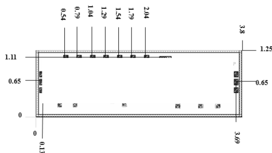
外形和端口尺寸( mm )
