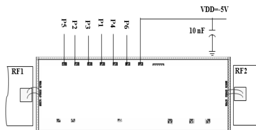
推荐装配图
