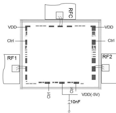
推荐装配图
