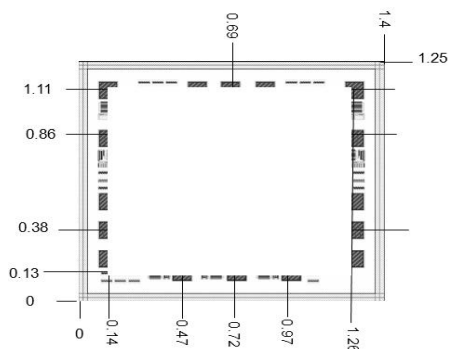
外形和端口尺寸 (mm)
