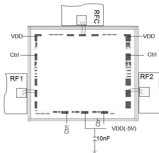
推荐装配图
