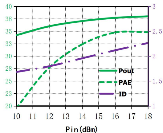
Pout (dBm)、PAE (%)、ID(A) vs. Pin,f=9.5GHz
