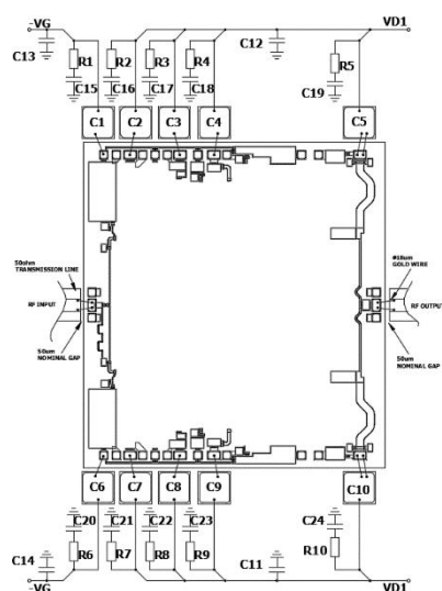
装配图
