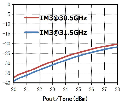
IM 3 (dBc)vs.Pout/Tone
