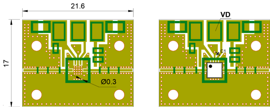
XT3098Q3 评估板
