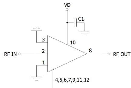
应用电路图
