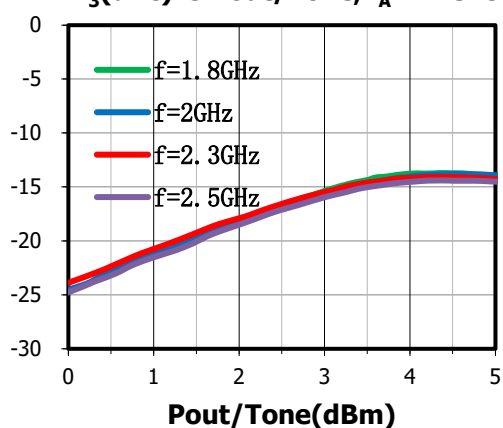
IM 3 (dBc) vs. P out /Tone, T A = +25°C
