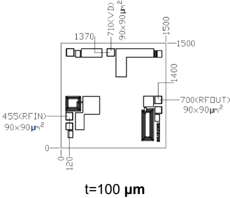
裸芯片外形尺寸( μm)
