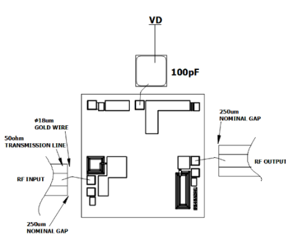
裸芯片推荐装配图
