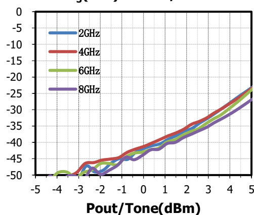
IM 3 (dBc)vs.Pout/Tone
