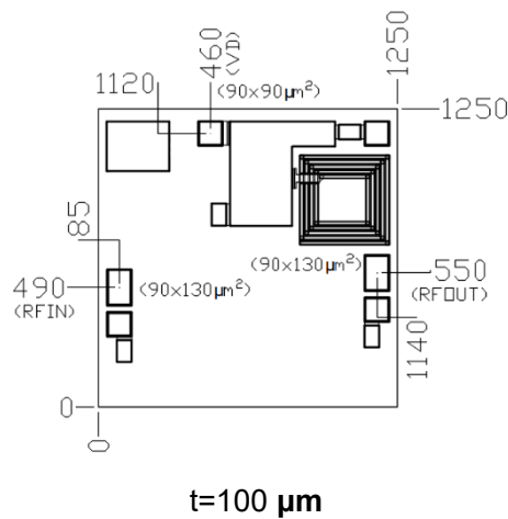
裸芯片外形尺寸( μm)
