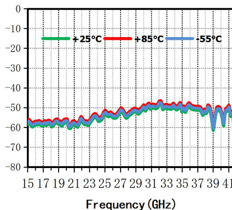
反向隔离(dB) vs. 温度
