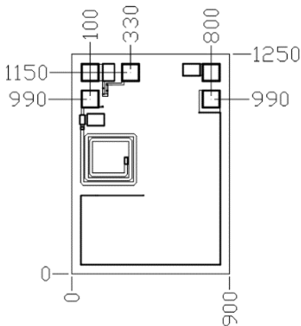
裸芯片外形尺寸图(μm)
