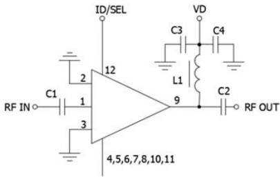
XT3089QP3 应用电路图
