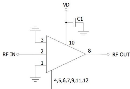
应用电路图
