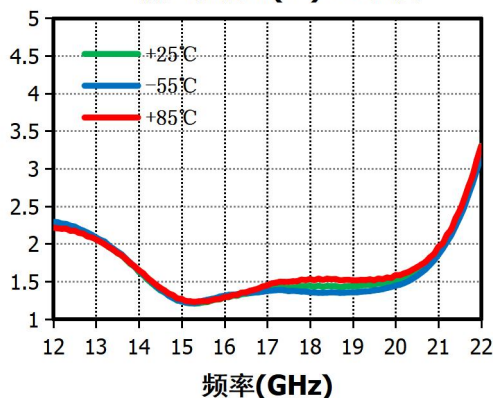
输入驻波比(:1) vs.温度
