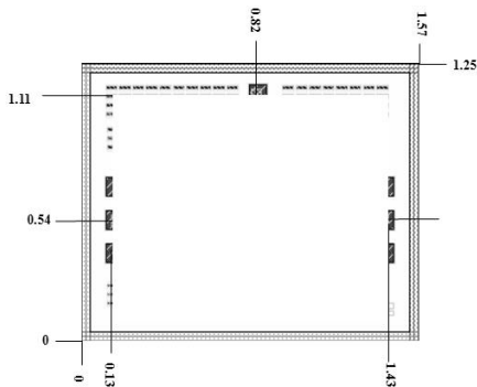
外形和端口尺寸 (mm)
