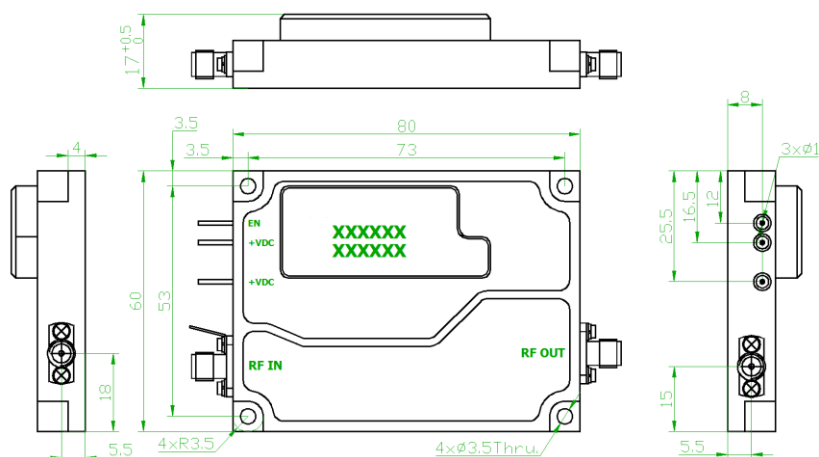
外形尺寸图 (mm)
