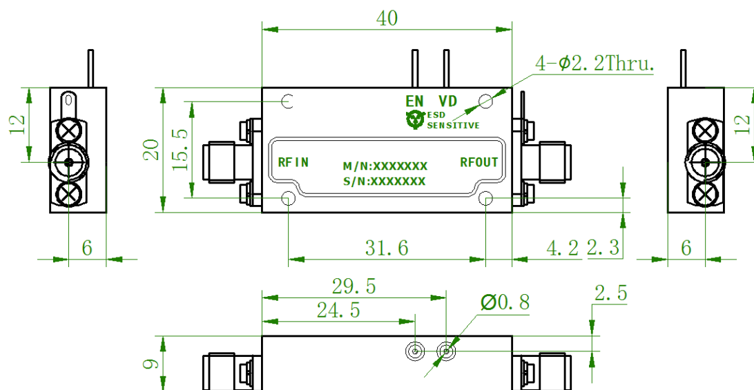
外形尺寸图(mm)
