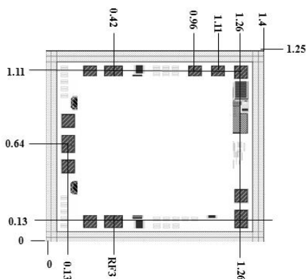
外形和端口尺寸 (mm)
