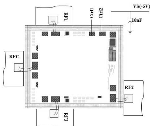
推荐装配图
