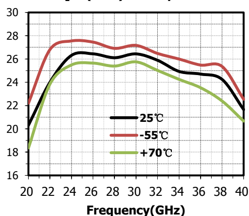
OP 1 dB(dBm)vs.Temperature
