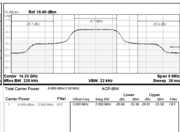
P_{OUT}=37\text{dBm} IDQ=2.45A
