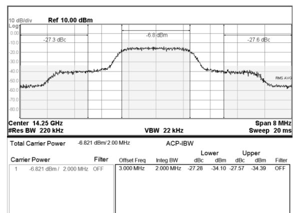
P_{OUT}=37\text{dBm} IDQ=2.45A
