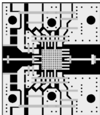
Evaluation PCB
